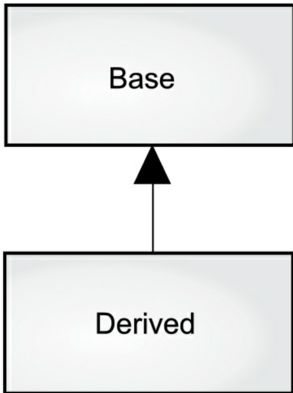
图 3: Inheritance-example
