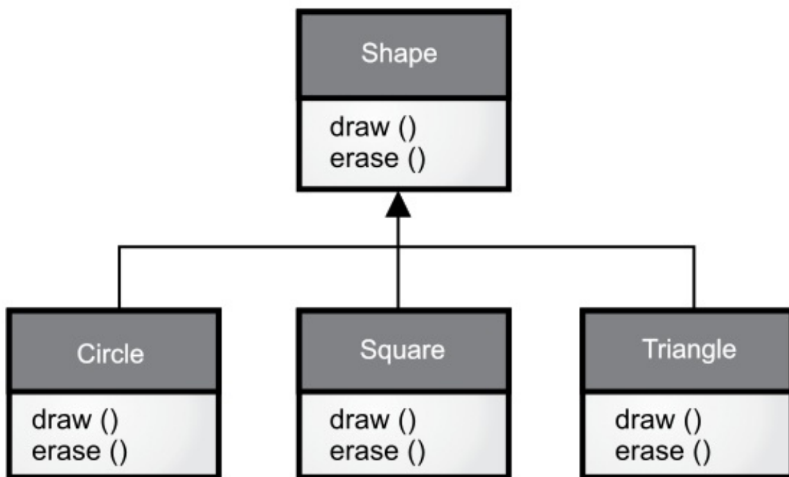
图 3: 类图
