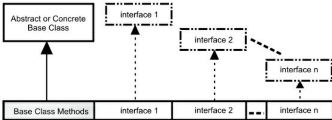
图 3: 类图
