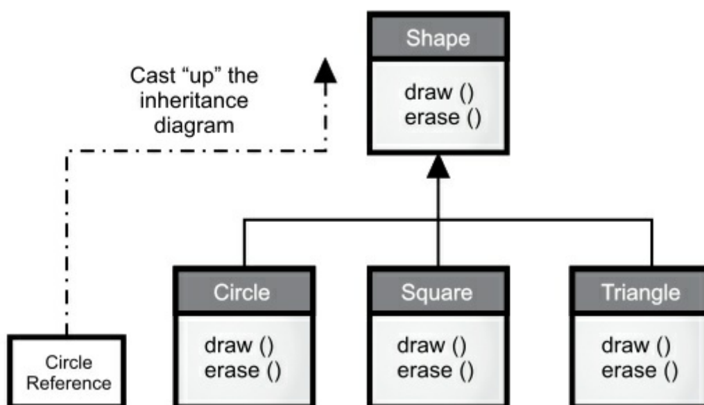
图 1: Wind 类图
