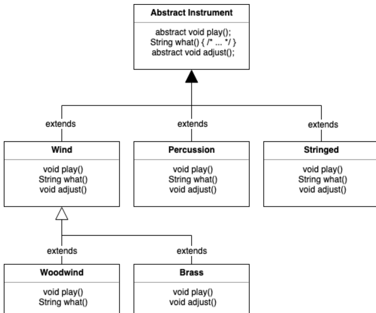
图 1: 类图
