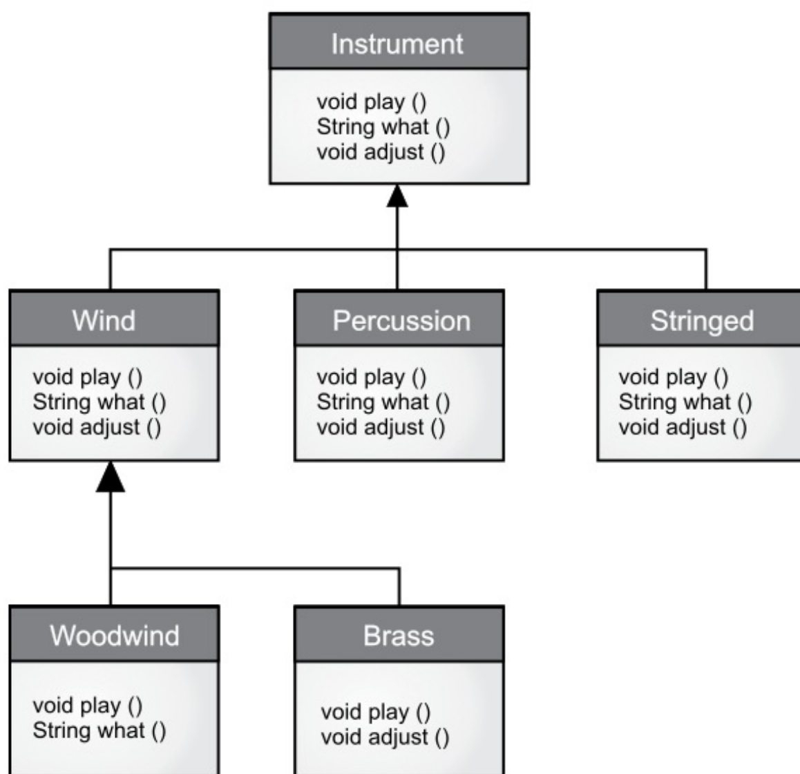
图 2: 乐器继承图
