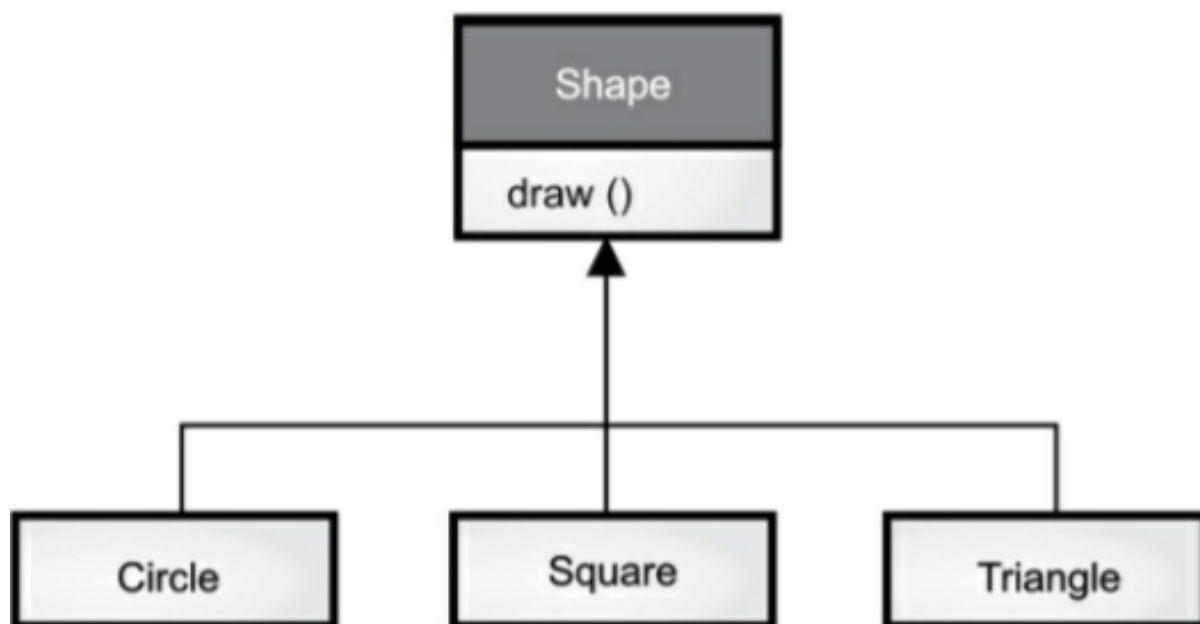
图 1: 多态例子 Shape 的类层次结构图
