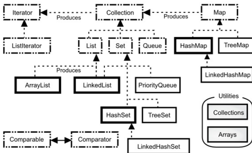
图 1: simple collection taxonomy
