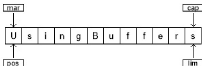
图 8: 1554546861836
