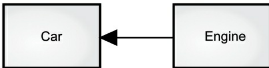
图 2: UML-example
